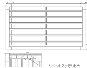
格子材断面図
