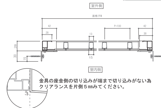
■横断面図
