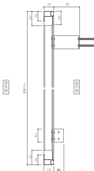
■縦断面図
