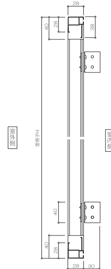
■縦断面図
