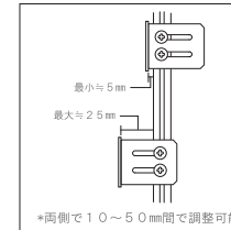
■金具の可動範囲 (面格子側)
