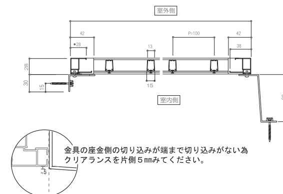
室外側
