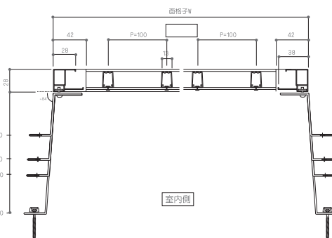
■横断面図
