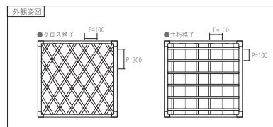
室外側
