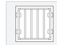
■格子出来寸法 開口W-20mm/開口H-10mm
