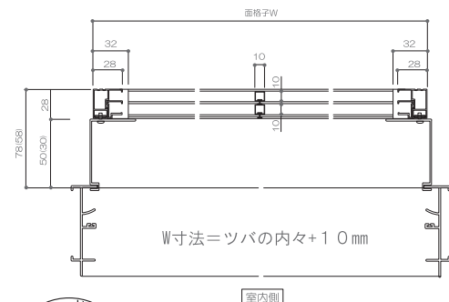
室内側
