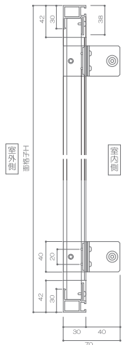
■縦断面図
