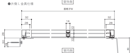
■横断面図
