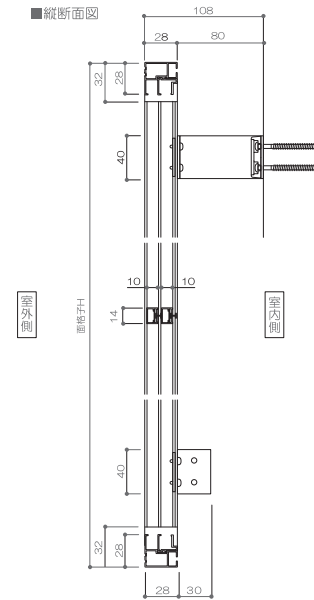
■縦断面図
