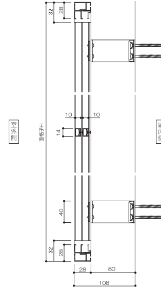
■縦断面図
