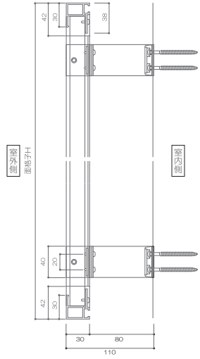
■縦断面図
